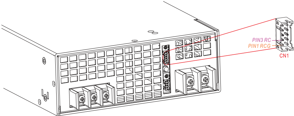
例2.2(A): 用外部电压
