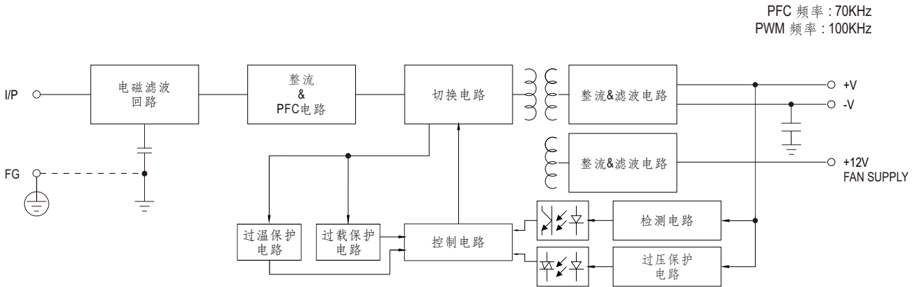
方框图
